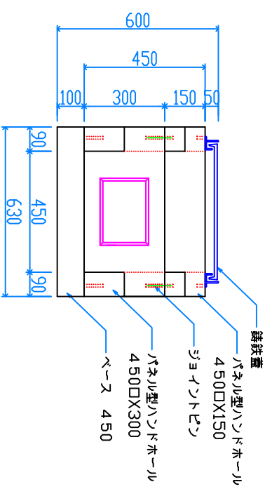
組立完成図
