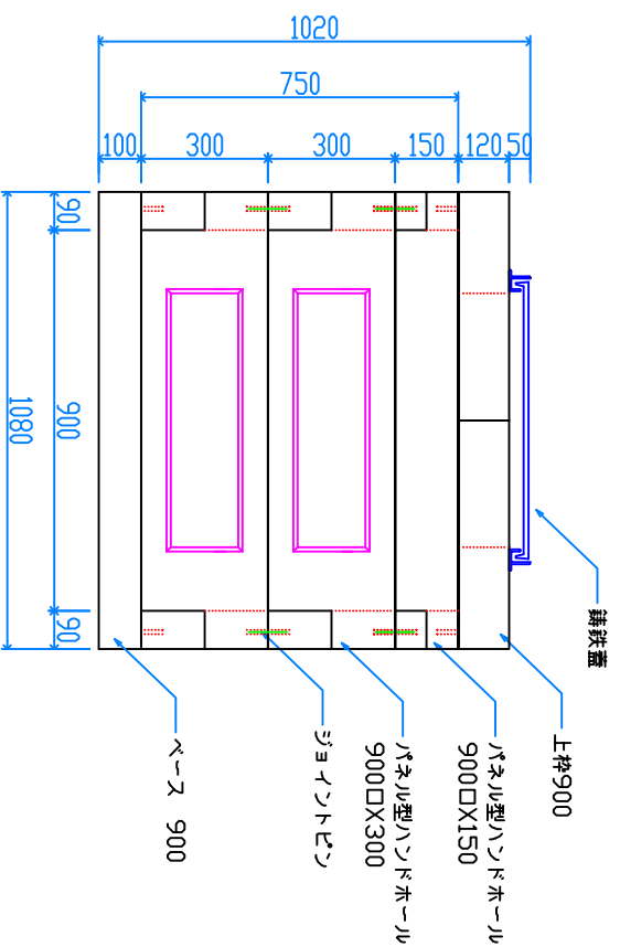
組立完成図
