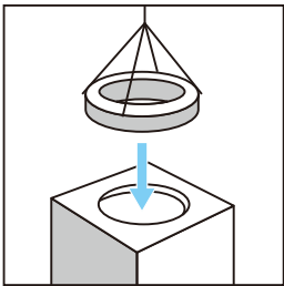
⑦CRを取り付けます。(4点吊り) CR・鋳鉄蓋固定用インサートに M12ボルトで固定
