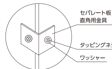
直角用補助セパ金具
