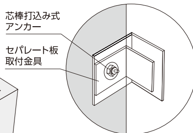
1000～1500用セパ金具
