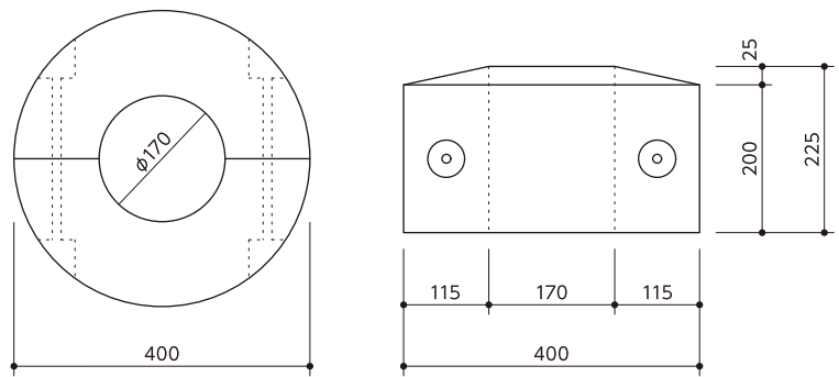
図面はAタイプです。(単位:mm)
