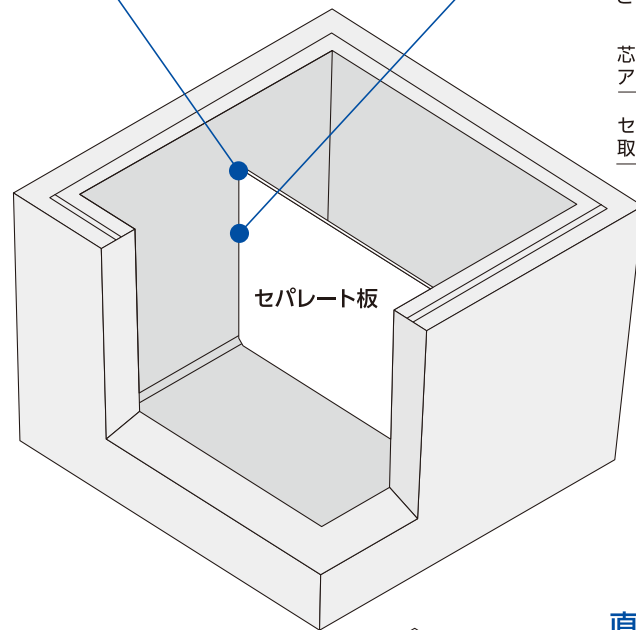
600～900用セパ金具
