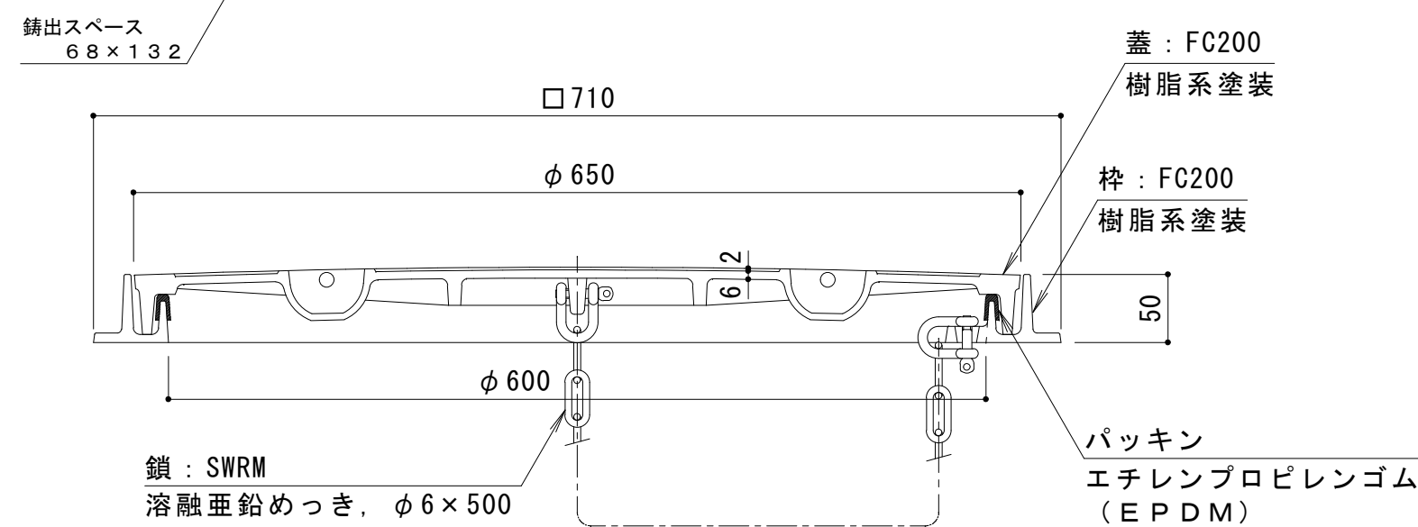
A-A断面図
