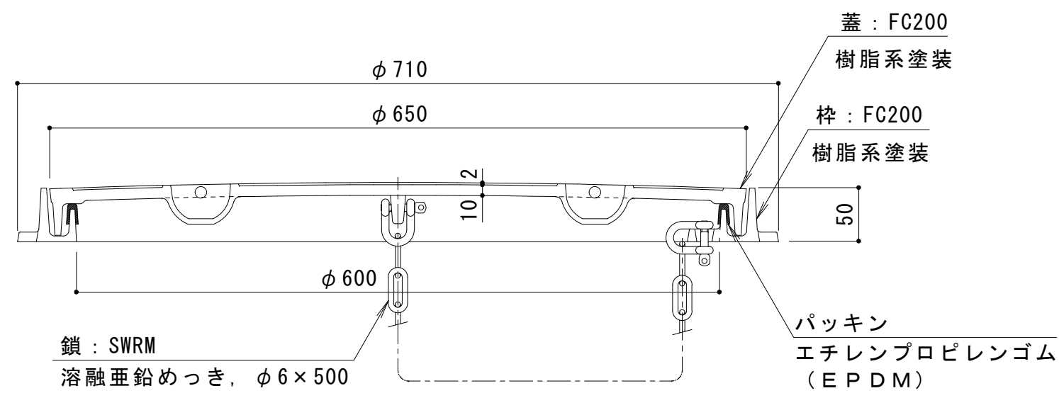
A-A断面図
