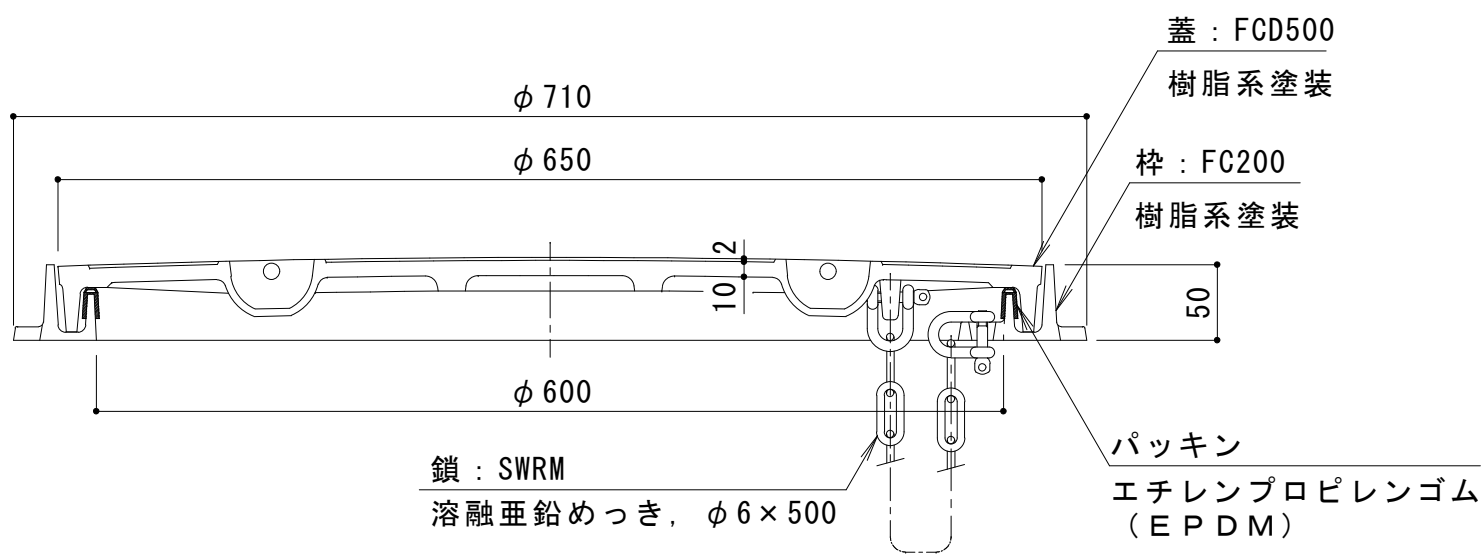
A-A 断面図
