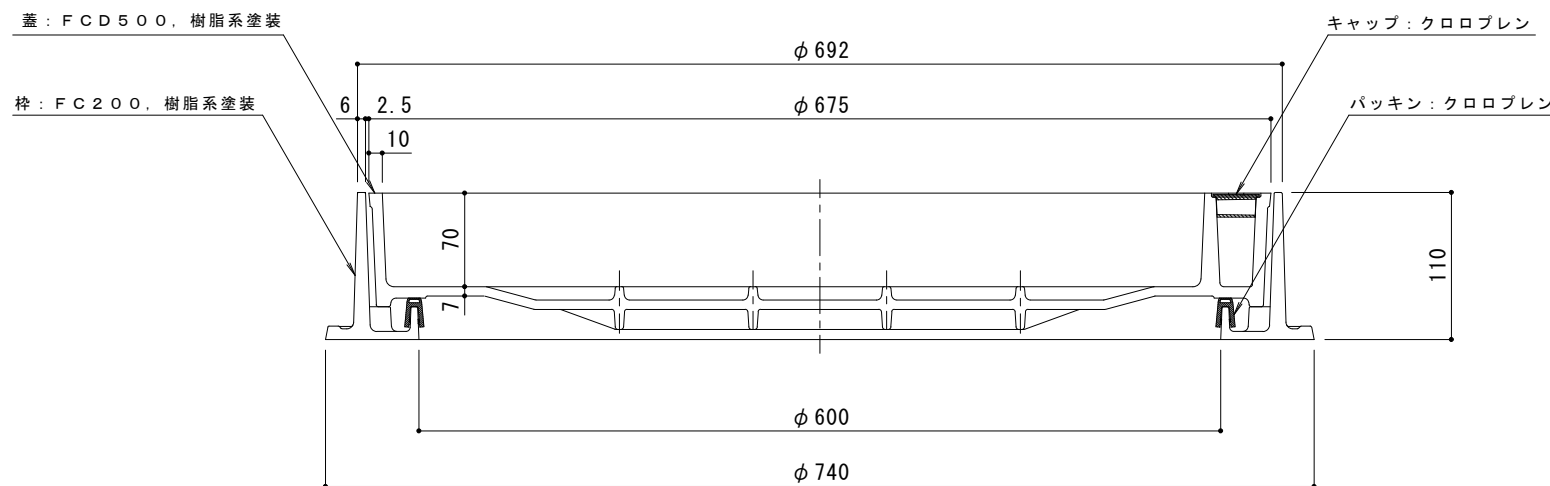
A-A断面図 S=1:4
