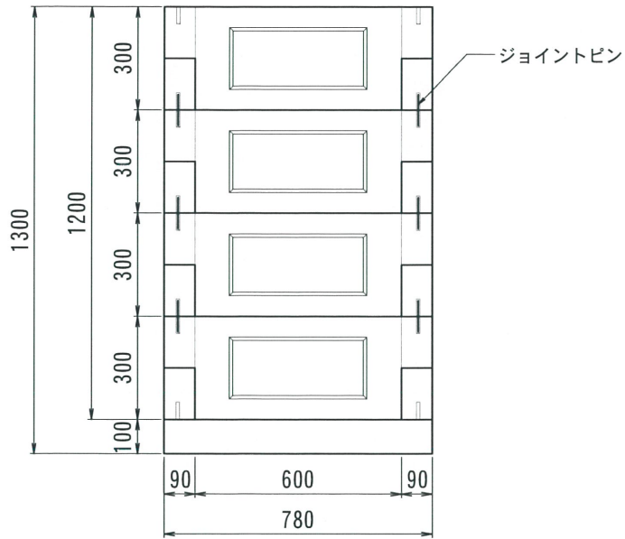
側面図
