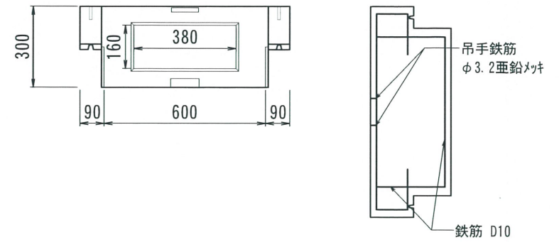
ハ° 衤型600 H-300
